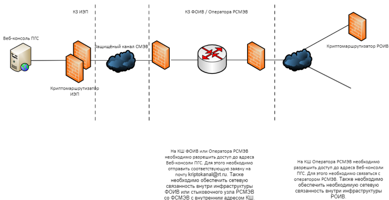
Рисунок — Схема оформления доступа к серверу ПГС
